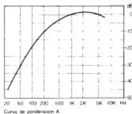
Curva de ponderación A
