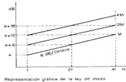
Representación gráfica de la ley de masa
